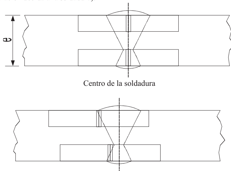
Zona de alteración debida a la soldadura
