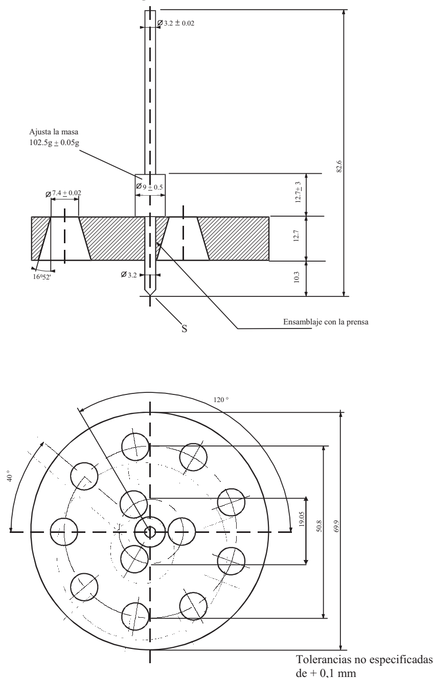
Figura 1 - Penetrómetro
